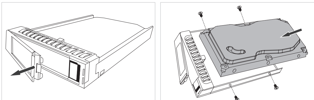
图3-2 安装硬盘
