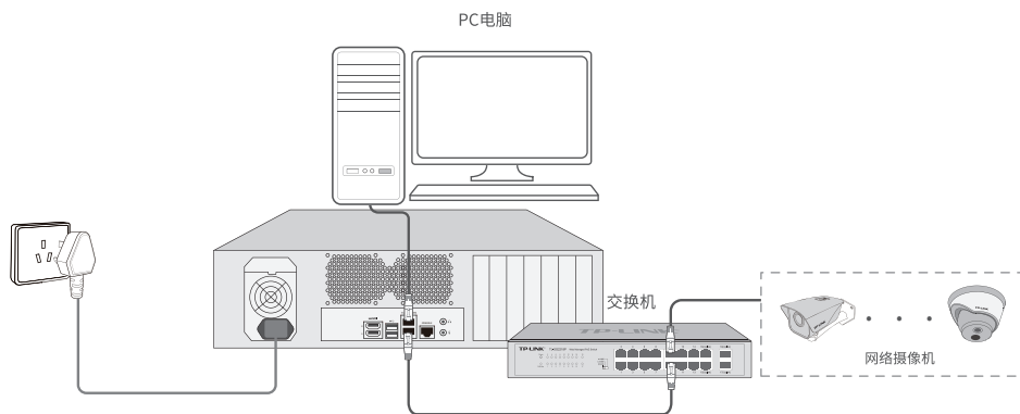
图3-3 NVS连接示意图
