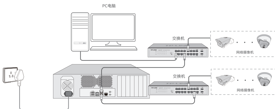
图3-4 NVS多址模式连接示意图
