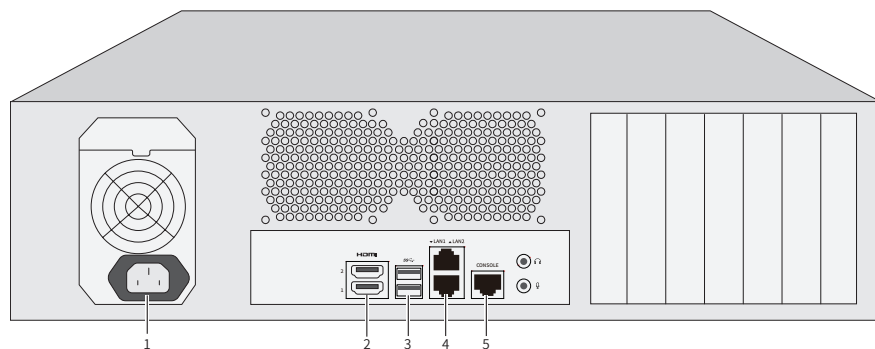
图1-3 TL-NVS7242-256后面板示意图
